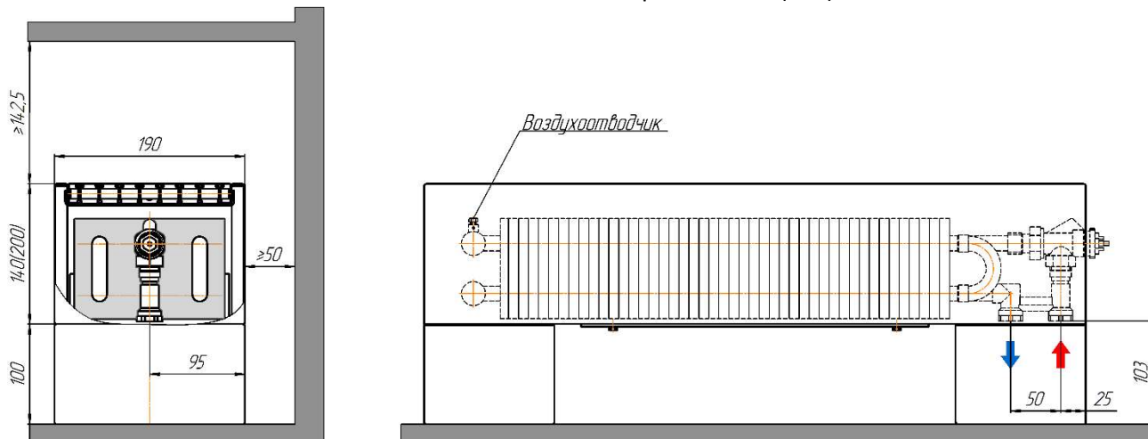
Монтажная схема ZOLTER Compact 190.250(300) U
