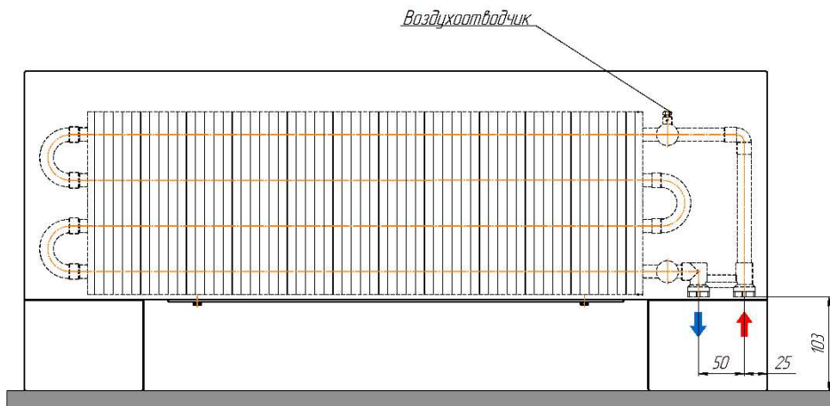
Монтажная схема ZOLTER Compact 140.250(300) UT
