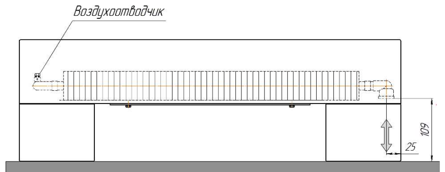
Монтажная схема ZOLTER Compact 140.110 UT
