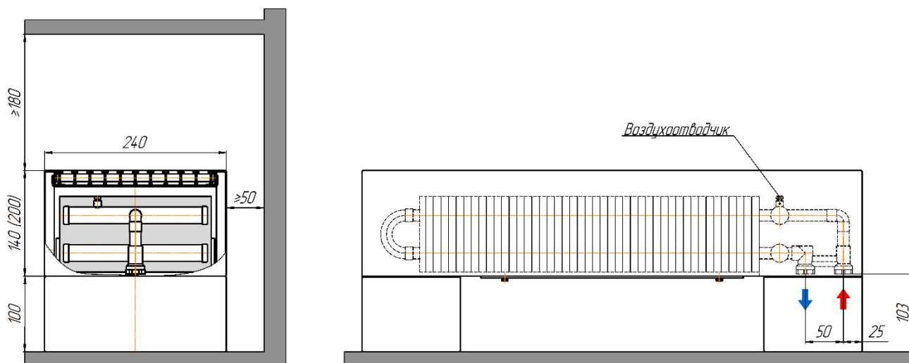
Монтажная схема ZOLTER Compact 240.140(200) U
