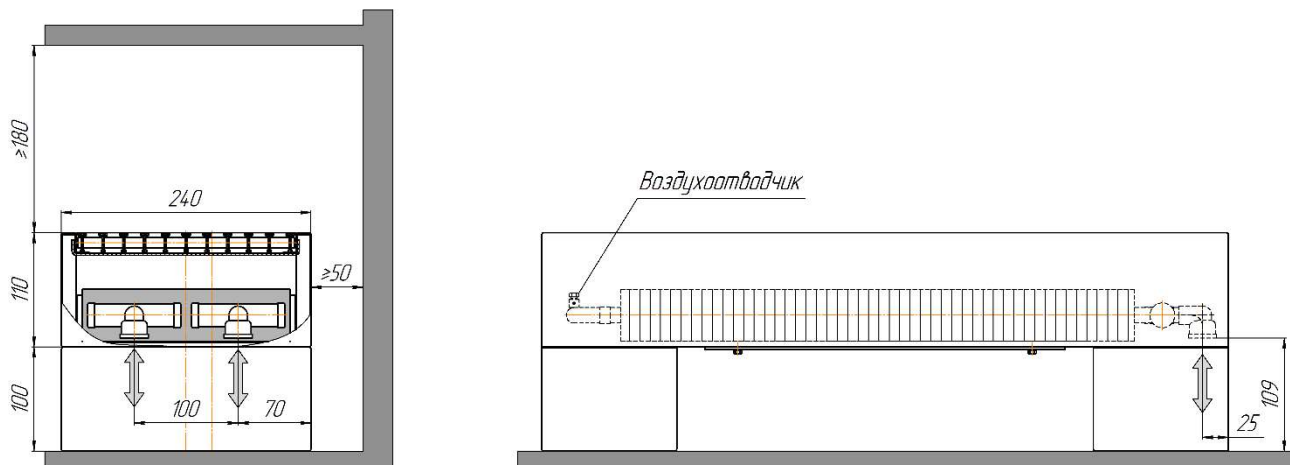
Монтажная схема ZOLTER Compact 240.110 UT
