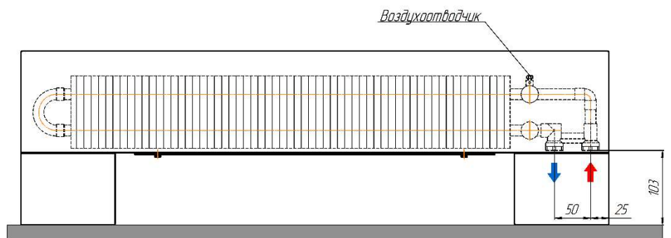
Монтажная схема ZOLTER Compact 140.140(200) U
