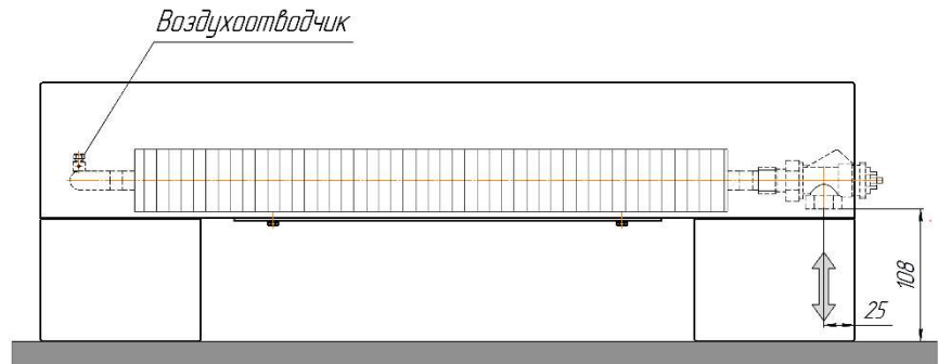
Монтажная схема ZOLTER Compact 140.140(200) U
