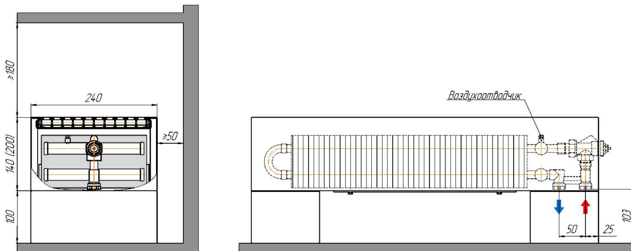
Монтажная схема ZOLTER Compact 240.250(300) U
