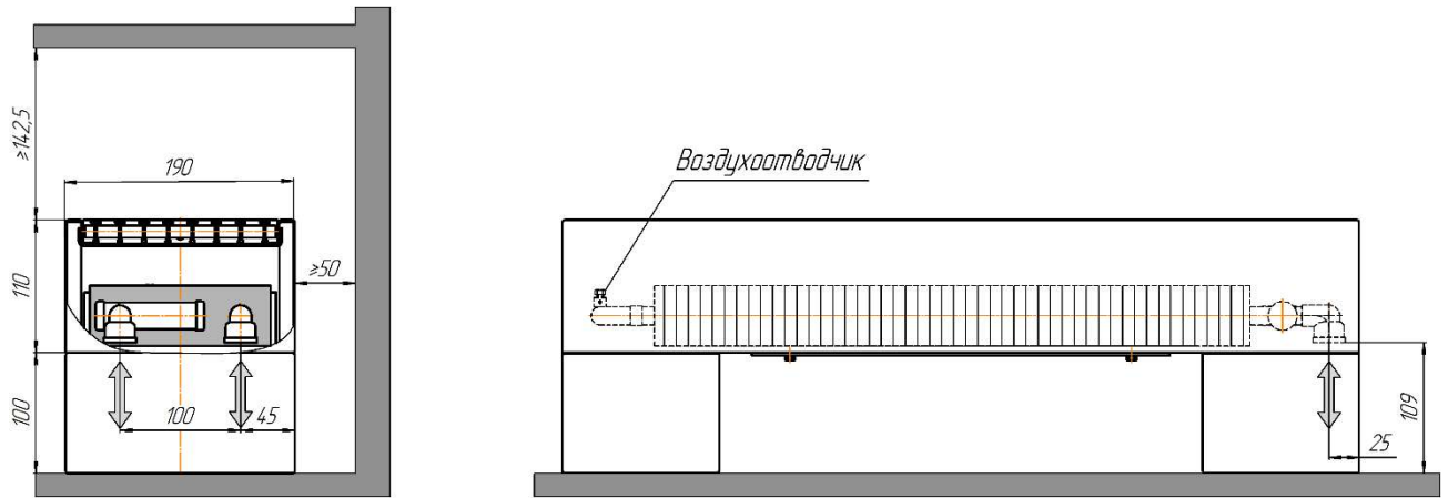
Монтажная схема ZOLTER Compact 190.110 UT
