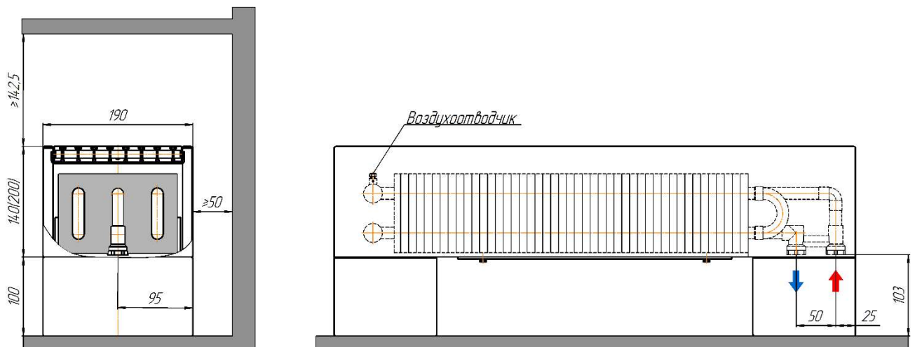
Монтажная схема ZOLTER Compact 190.140(200) U
