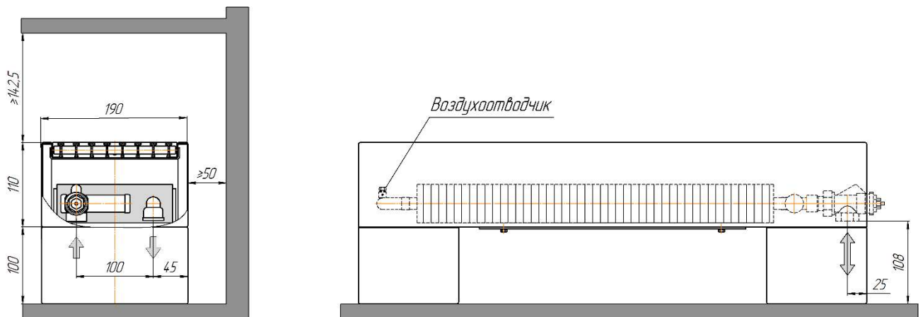
Монтажная схема ZOLTER Compact 190.140(200) U
