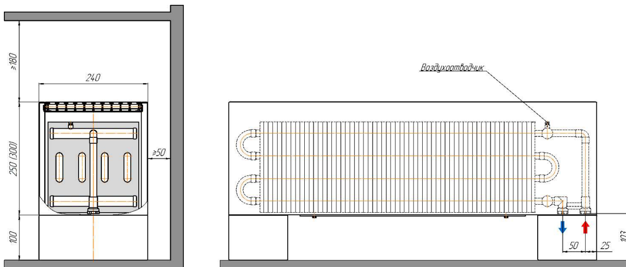
Монтажная схема ZOLTER Compact 240.250(300) U
