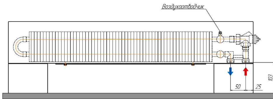
Монтажная схема ZOLTER Compact 140.250(300) U
