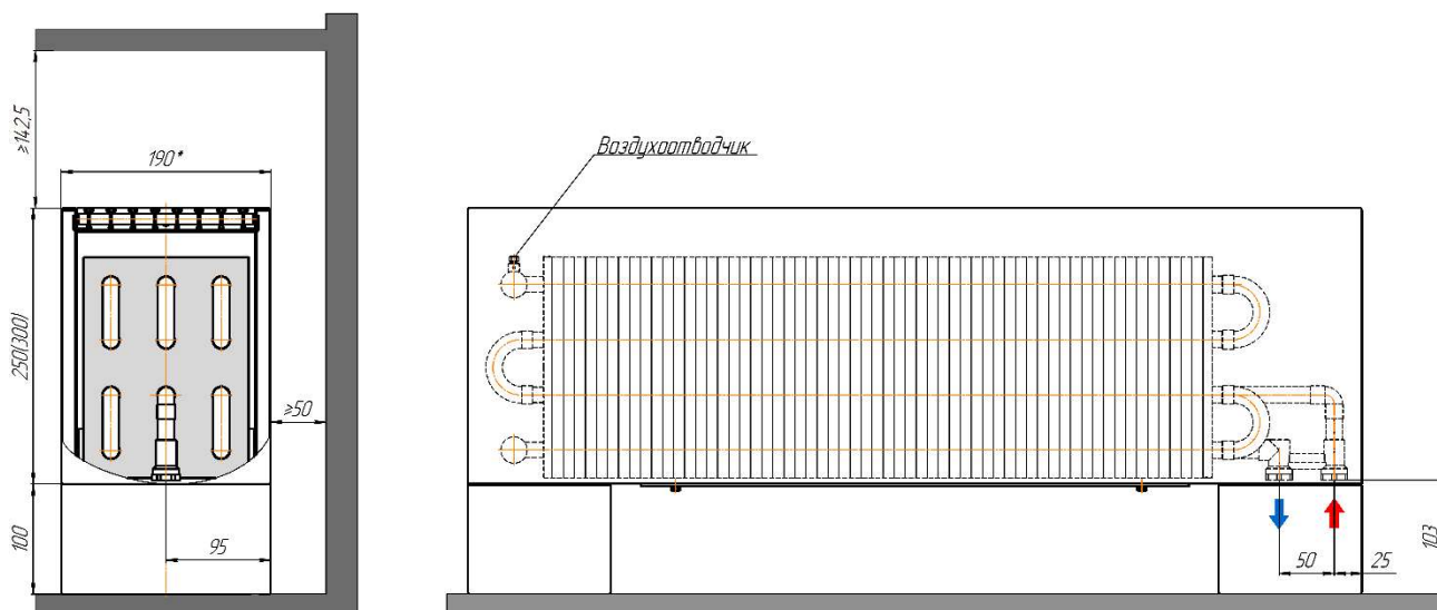
Монтажная схема ZOLTER Compact 190.250(300) UT
